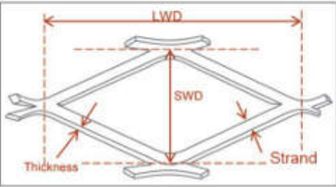
Key Dimensions 关键尺寸图
